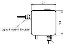
Elektronikbox 94x94x56mm
