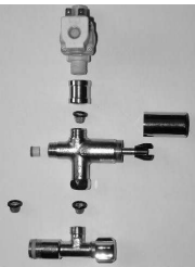
Magnetventil Mischung über DMS-Mischer zur Direktmontage auf Eckventil(bauseitig) mit RüVe in KW/WW
