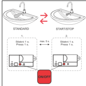
Veränderungsmöglichkeit Standard-Programm zu Start/Stop-Programm durch optionale Fernbedienung (Remote-Control)
