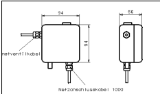
Elektronikbox 94x94x56mm
